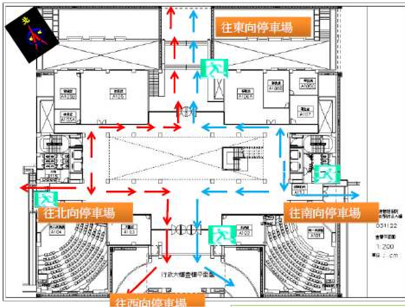
行政大樓 1 樓 逃生平面圖
