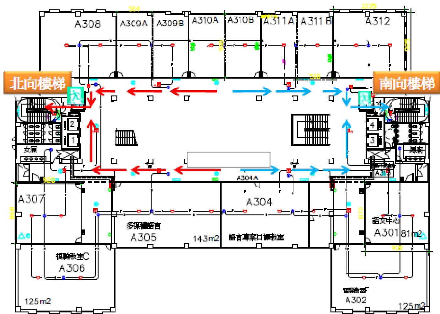
行政大樓 3樓 逃生平面圖
