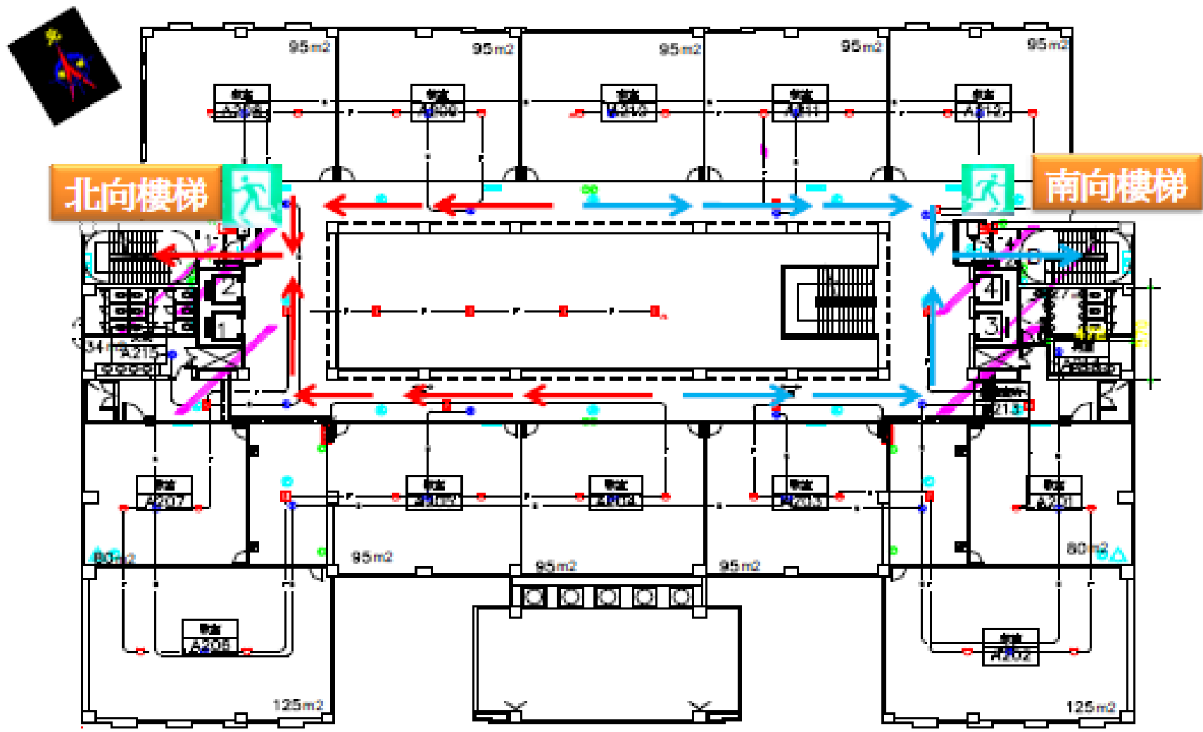
行政大樓 2 樓 逃生平面圖
