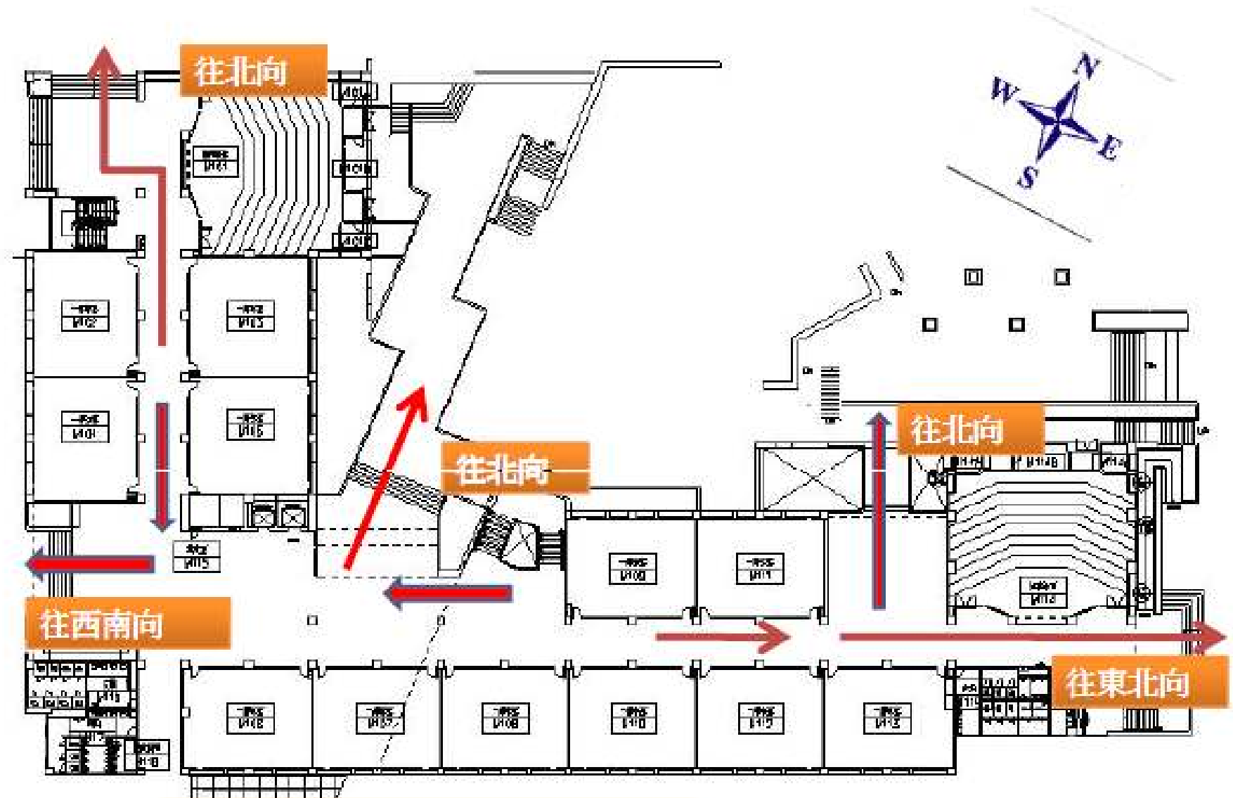
管理大樓一樓消防逃生平面配置圖
