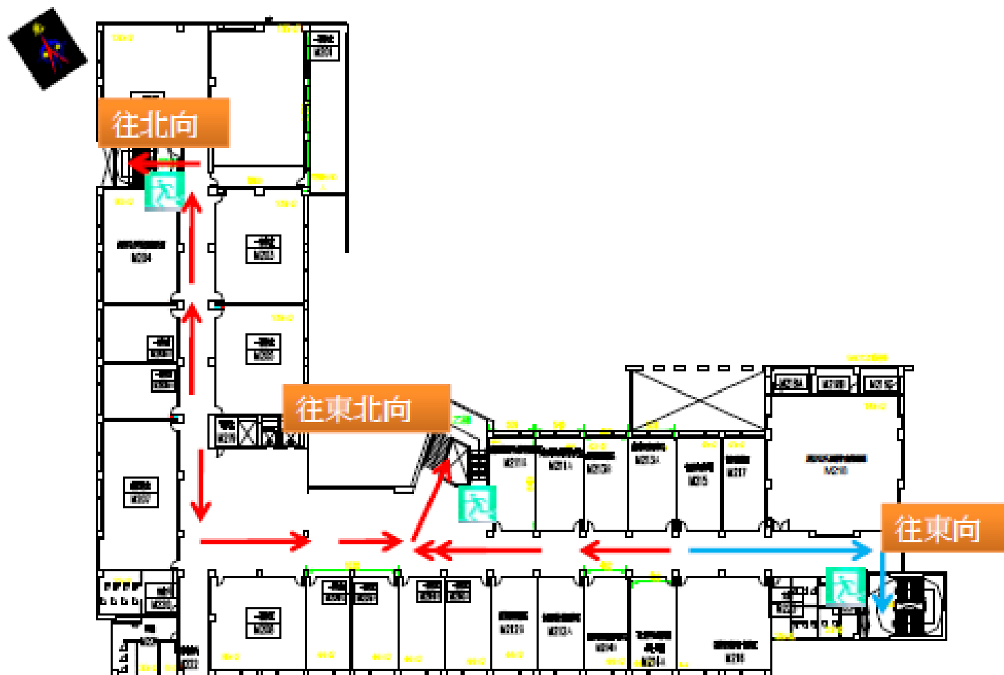
管理大樓二樓消防逃生平面配置圖
