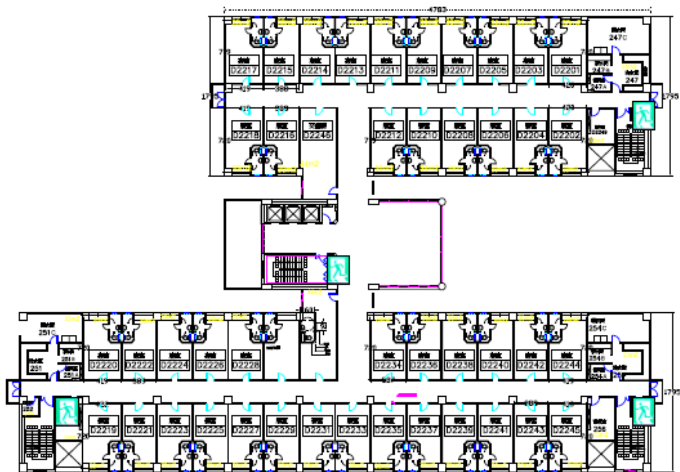
女生宿舍-貳樓逃生平面圖 ● 現在位置 → 逃生方向
