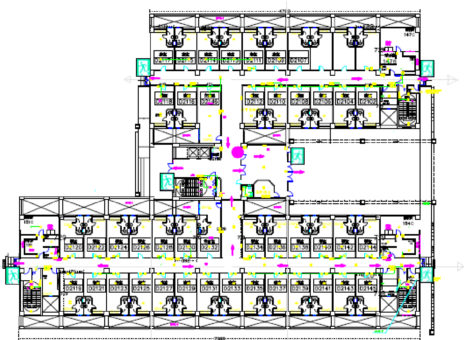
女生宿舍-壹樓逃生平面圖 ● 滅火位置 → 逃生方向
